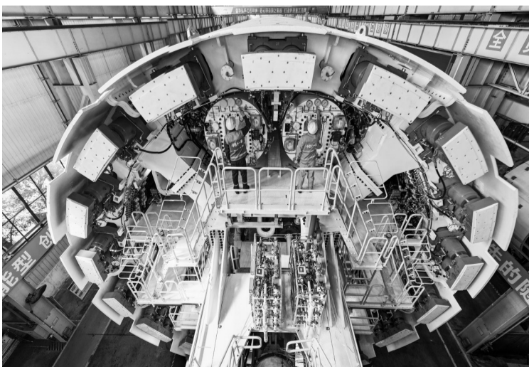
11月9日,由中铁十一局和铁建重工联合打造的“永庆号”盾构机在湖南长沙顺利下线。图为11月9日,在铁建重工长沙第一产业园,工人在调试“永庆号”盾构机(无人机照片)。
