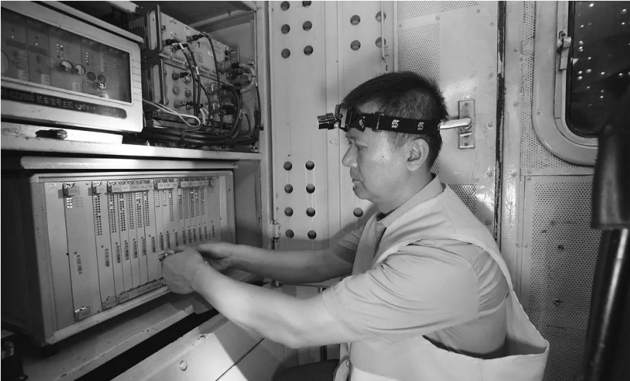
火车“黑匣子”学名叫列车运行监控装置,它主要由监控主机、显示器、速度传感器等设备构成。铁路供图
