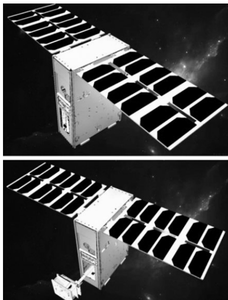
“天帆一号”两级展开过程示意图。
