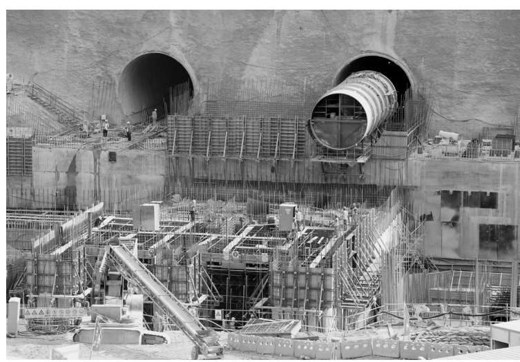
这是7月27日拍摄的新疆大石峡水利枢纽工程发电厂建设现场。据介绍,截至7月27日,新疆大石峡水利枢纽工程大坝已填筑至1500米高程,电站主要建筑物发电厂房、溢洪道、联合进水口等均按进度在紧张施工之中。新疆大石峡水利枢纽工程是国家节水供水重大水利工程,工程主要建设内容为挡水坝、溢洪道、引水发电系统等。新华社记者 房俊伟 摄
