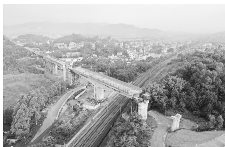
完成转体的南玉高铁跨黎湛铁路特大桥转体梁(5月24日摄,无人机照片)。5月24日凌晨,由中铁二局集团承建南玉高铁跨黎湛铁路特大桥成功转体57度。新华社发
