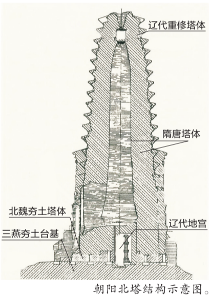
朝阳北塔结构示意图。
