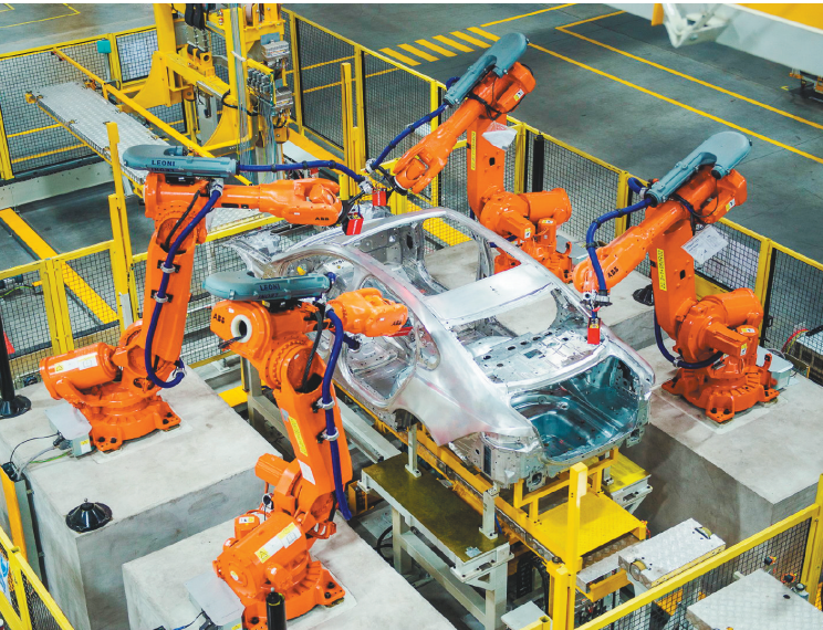
东风日产自动化生产线。
