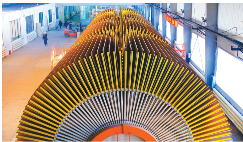
辽宁尼科达环保材料有限公司的全自动化生产线。本报记者 郑磊 摄
