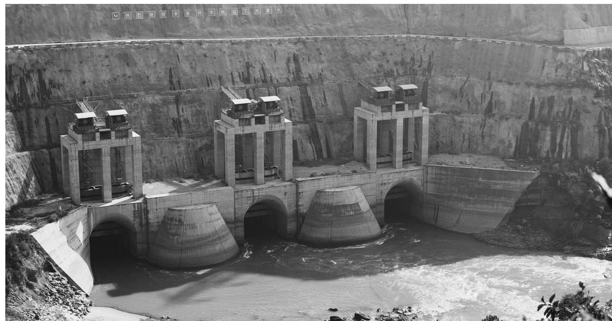
这是11月19日在巴基斯坦旁遮普省拍摄的卡洛特水电站导流洞闸门。 新华社发
