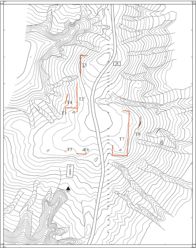
牛河梁遗址第一地点主要遗迹分布示意图。
