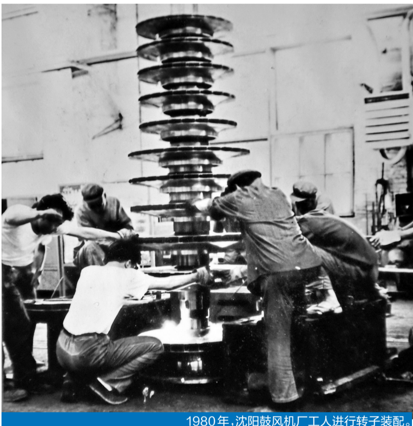
1980年,沈阳鼓风机厂工人进行转子装配。
